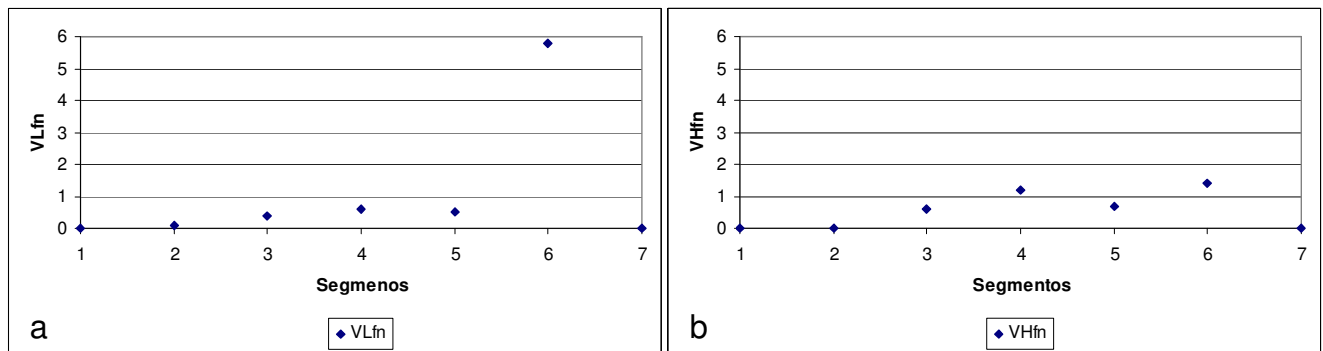
Figura 7: Volumes de água doce disponíveis nas estofas de maré baixa (a) e maré alta (b) ( 10^6m^3 ) por segmentos, respectivamente.
