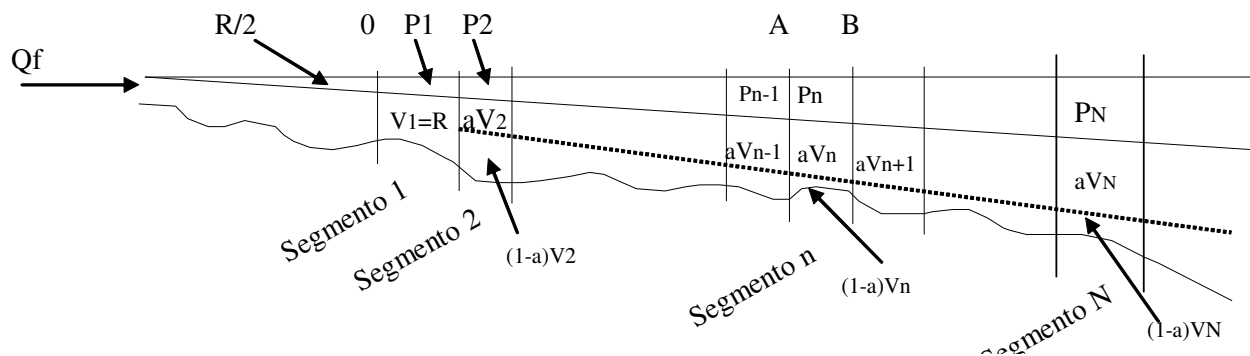
Figura 3: Modelo hipotético da metodologia de Dyer e Taylor (1973). P_n e V_n denotam os volumes do prisma de maré e de maré baixa de um segmento genérico n ( a é o parâmetro de mistura), (1-a)V_n é o volume na maré baixa disponível para mistura na maré alta, R é o volume de água fluvial descarregado no estuário durante um período de maré ( T = 43082 segundos para maré semi-diurna), A e B são segmentos hipotéticos.
