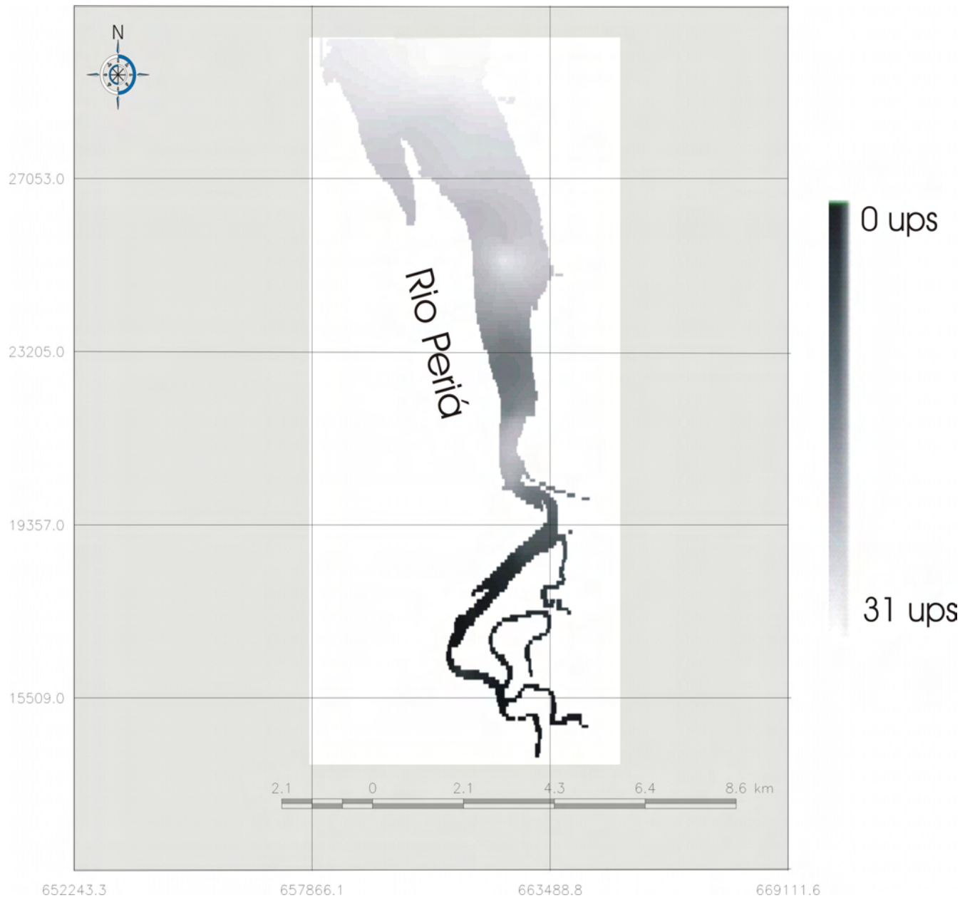
Figura 2: Salinidade do Estuário durante a maré cheia.
